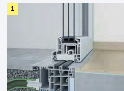
1 | Nullbarriereschwelle: Magnet-Dichtungsprofile dichten die geschlossene Balkontür sicher ab.
